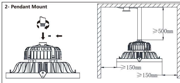
2- Pendant Mount
