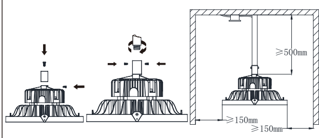
2- Pendant Mount
